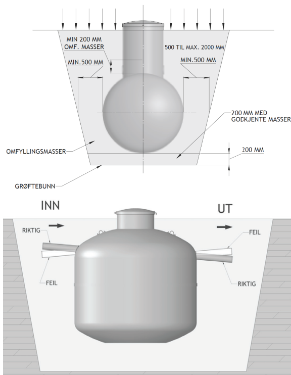
Figur 8: Standard installasjon. For å unngå motfall inn og ut av tanken, er det viktig med god komprimering under rørslutningene
