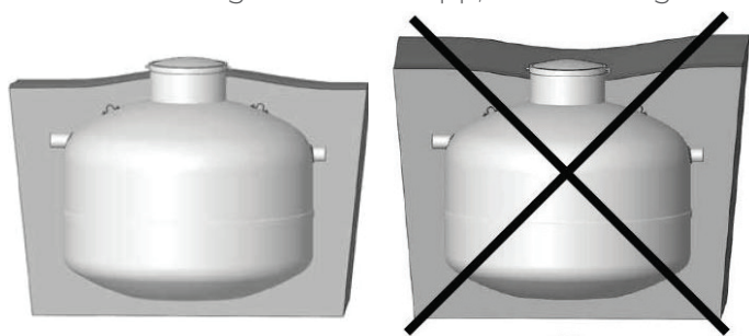
Figur 4: Riktig avrenning.
