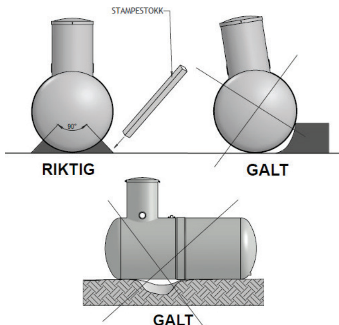
Figur 7: Pakking av fyllmassene under tankens nederste kvartsirkel.
