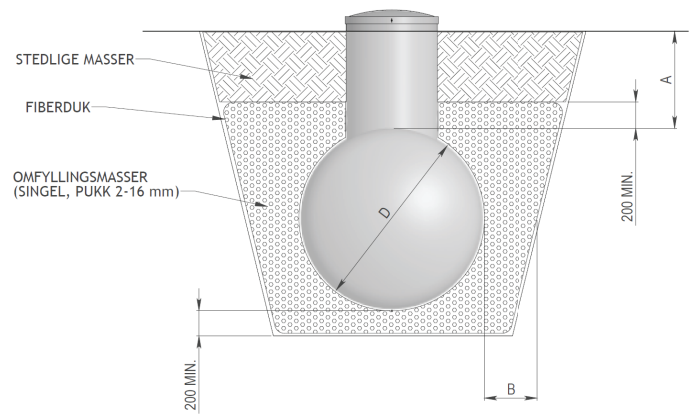
Figur 2: Installasjon i løse masser. Se også tegning A 8290d Kilde: VPI - Transport- og nedleggingsanvisning for tank i glassfiberarmert polyester (GRP).
